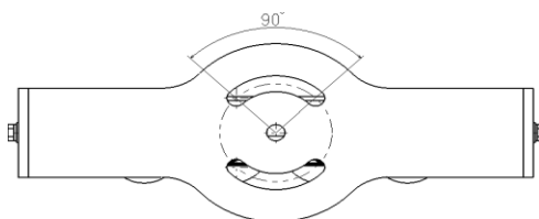
アームの回転範囲 / rotation range of ARM
