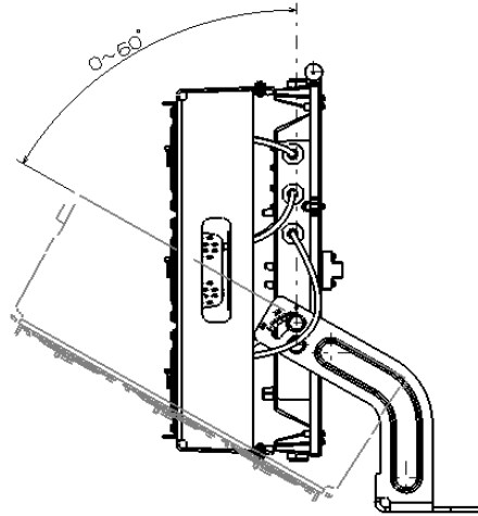
下向きアーム灯具の回転範囲 / Rotation range of downward arm lamp
